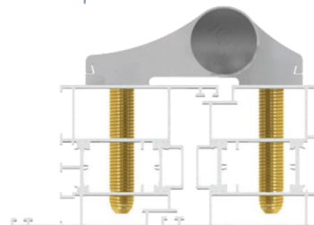
Самонарезающие болты для тёплых профилей с термовставками
