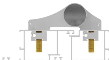
Закладные с винтами для холодных профилей
